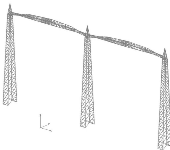
Fig. E3 – Portale
